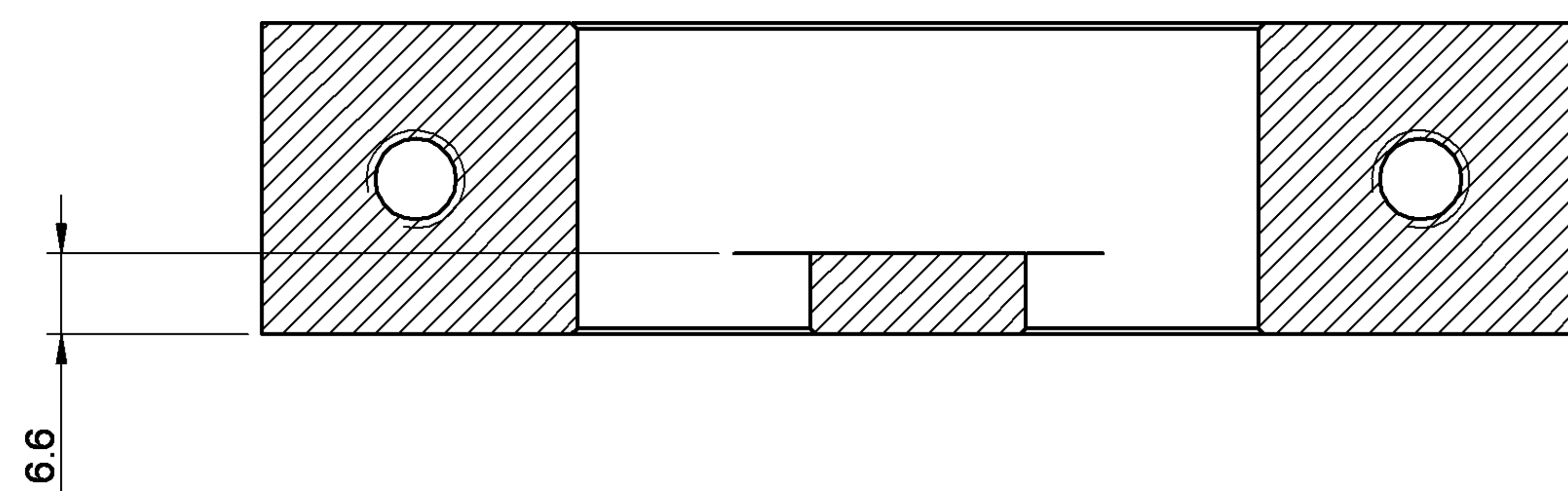
SECTION A-A
